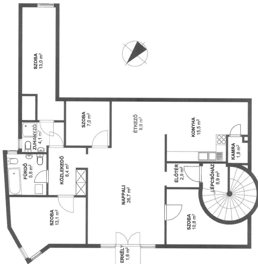
Tetőtéri alaprajz
